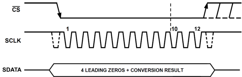
时序图
