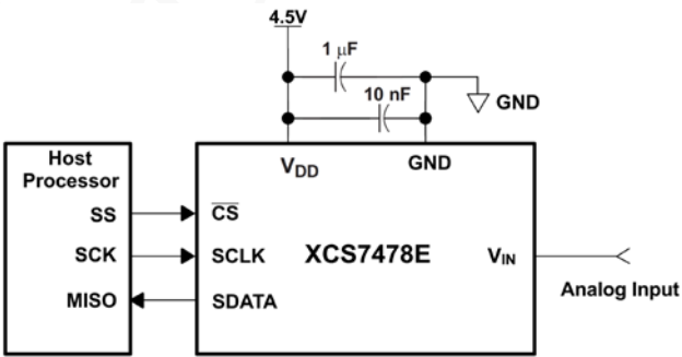
电路连接图
