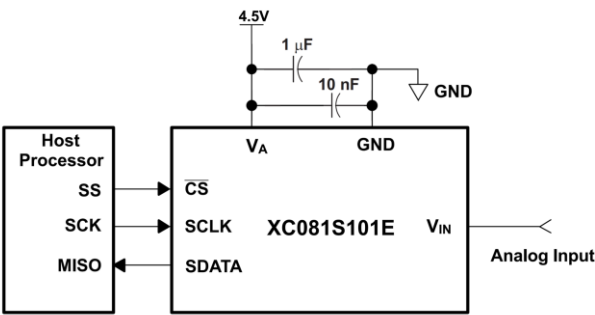
电路连接图
