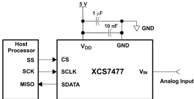
电路连接图
