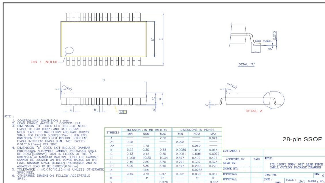
图 2 SSOP28 封装信息
