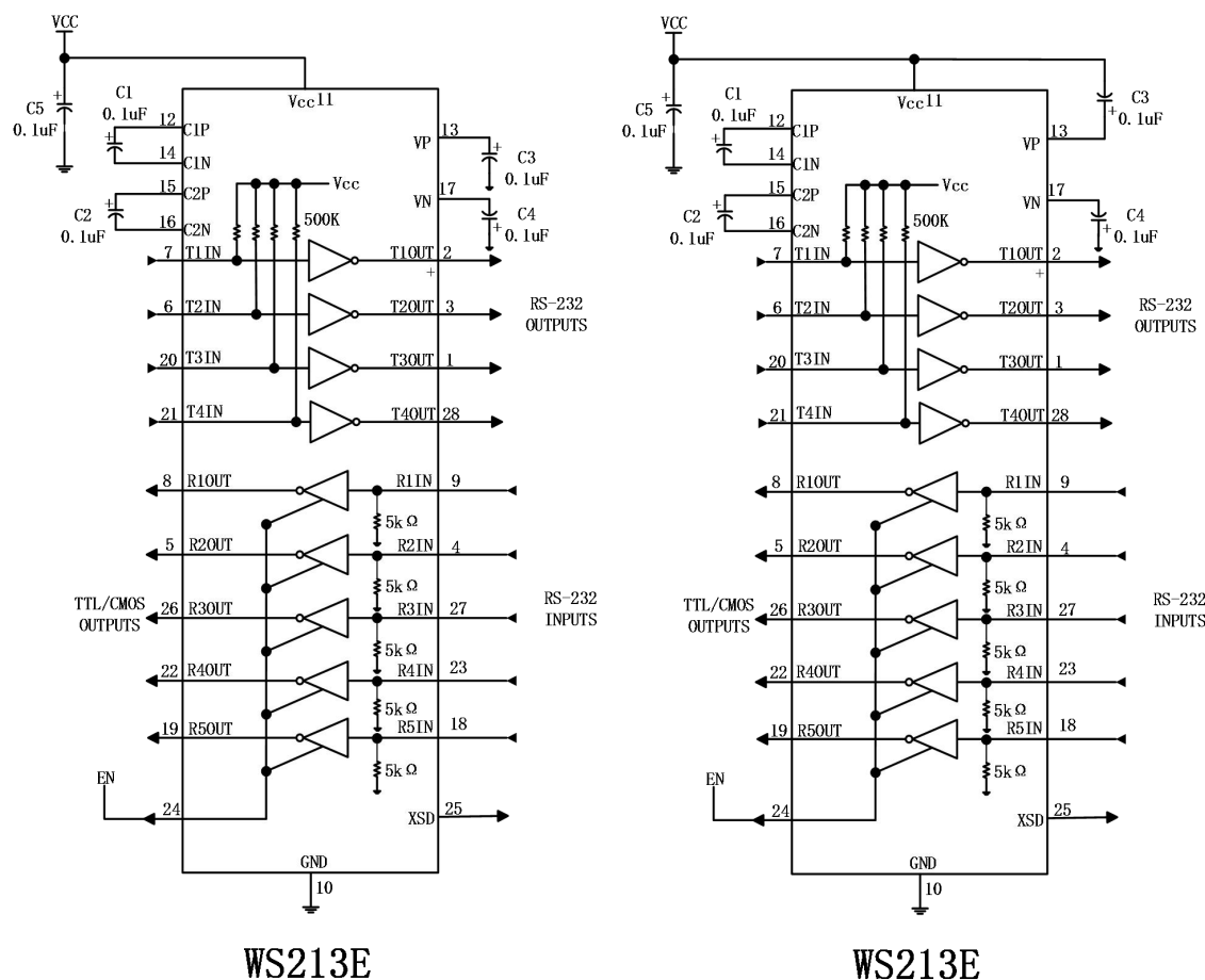
图 1 WS213E 典型外围应用电路
