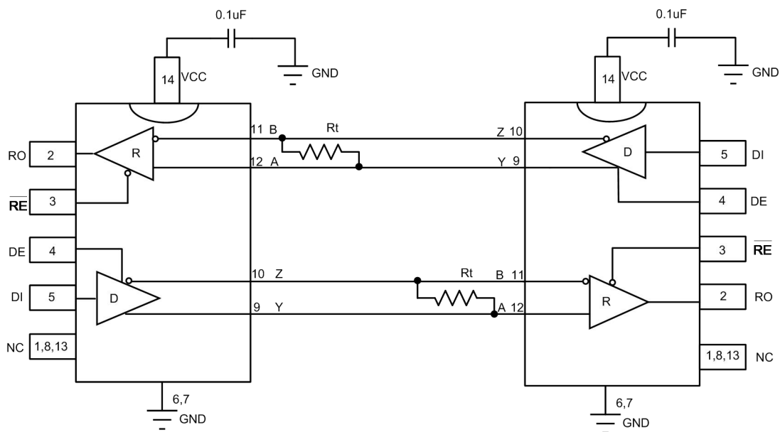
图 10 GB491 典型全双工工作电路
