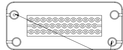
Key Feature/定位柱 (99X-35X-2001/99X-35X-5067/99X-353-6067)
