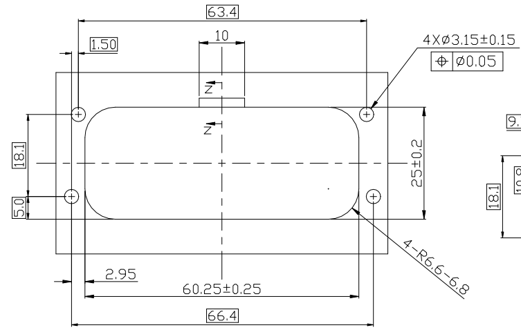
Mounting Panel Size (Maximum Gauge5.0mm) 安装面板尺寸(最大厚度5.0mm)
