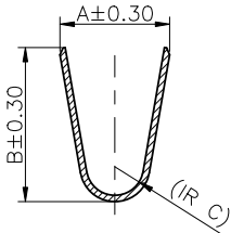
SECTION:G-G
