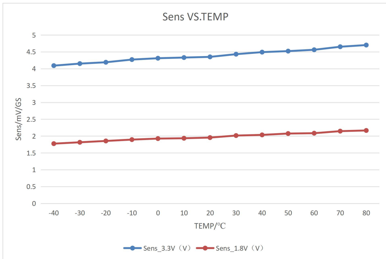
Sens VS.TEMP
