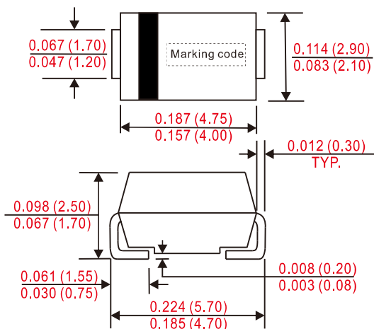
DO-214AC(SMA)
