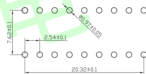
PCB开孔
