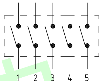
电路图
