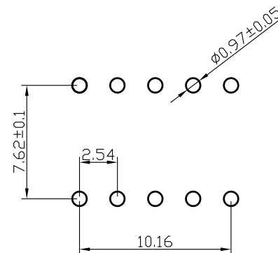
PCB开孔
