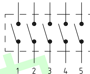
电路图
