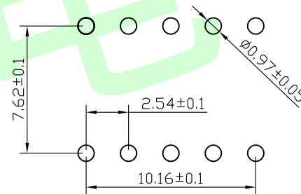
PCB开孔
