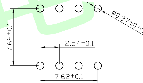
PCB开孔
