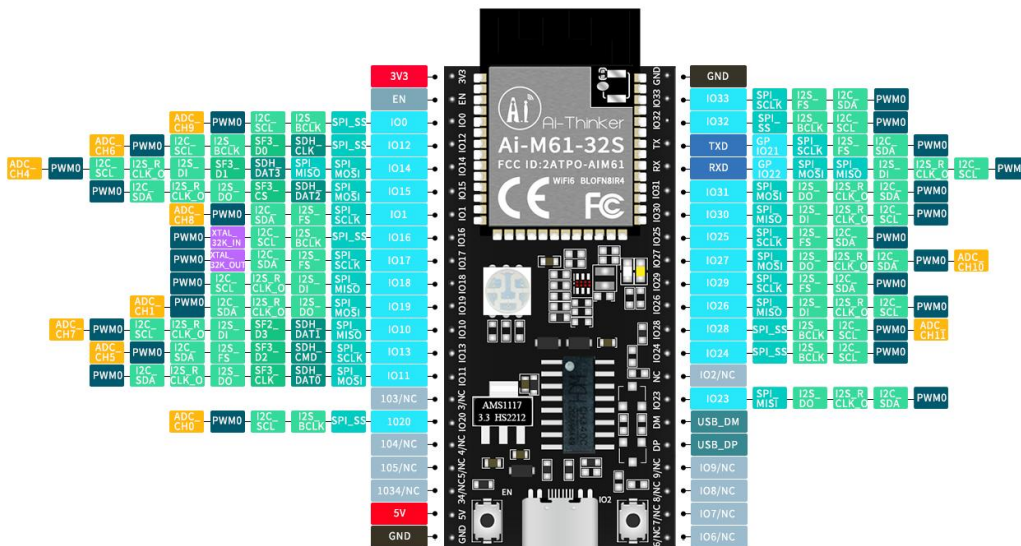
Ai-M61-32S开发板管脚图示
