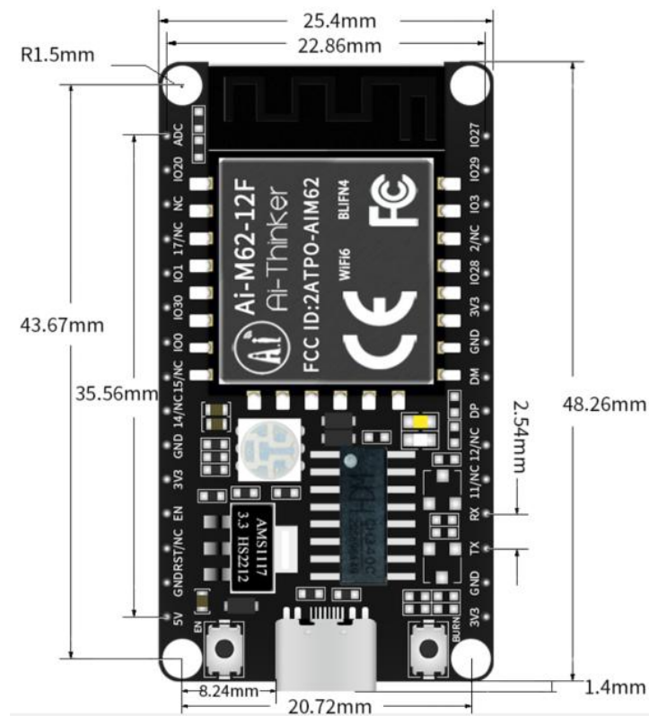
图 4 尺寸图
