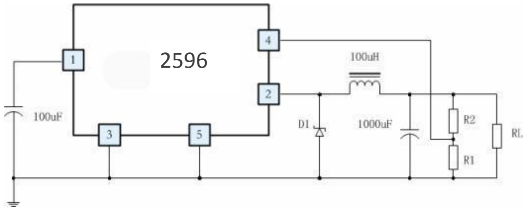
图 1 LM2596T-ADJ 应用图例
