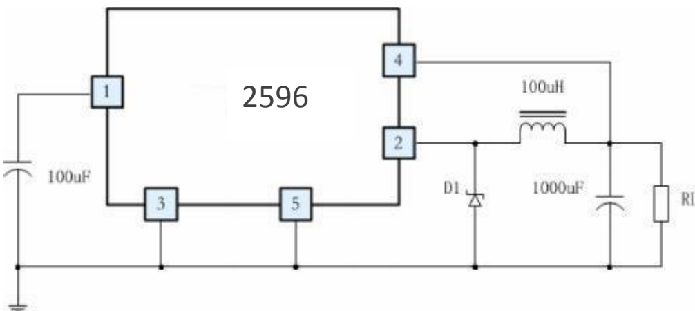
图 2 LM2596T-5.0V/12.0V 应用图例
