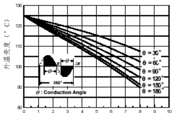
图五、通态电流---外壳温度
