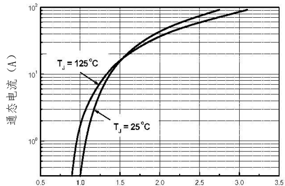
图二、通态电压
