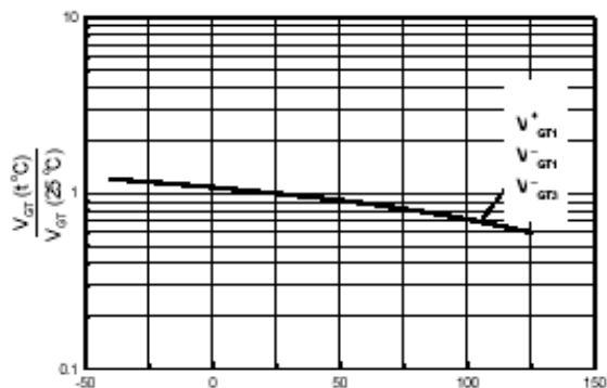
图三、门极触发电压-----结温
