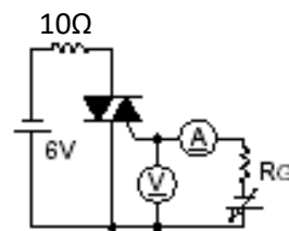
测试方式 III
