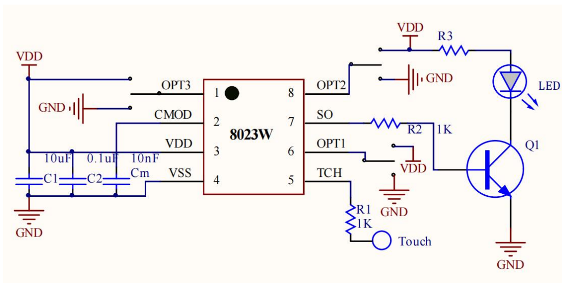
标准应用电路(VDD=2.5~5.5V)
