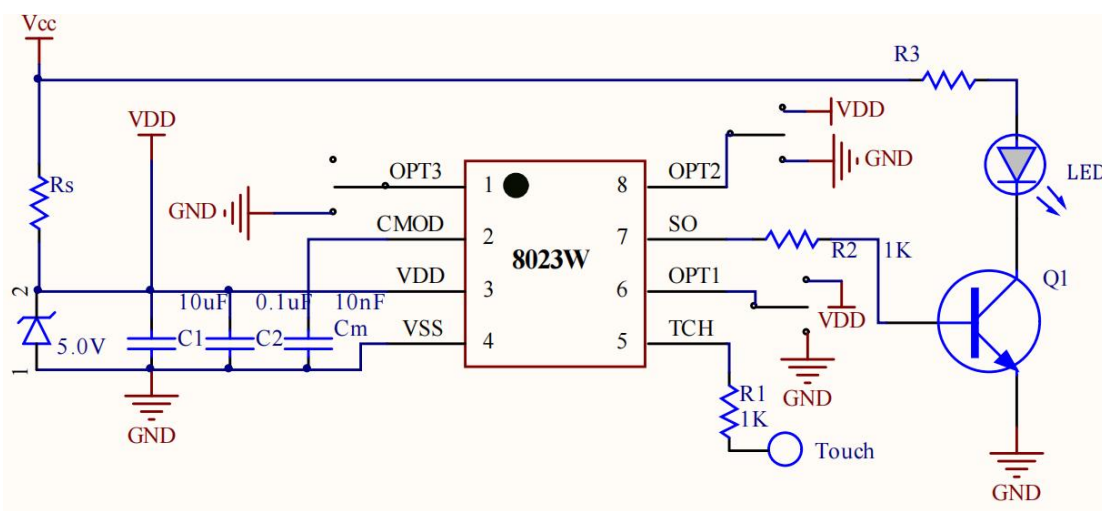
直流高压供电应用电路( V_{CC} > 5.5V )
