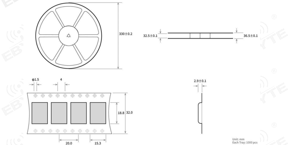
图 10 批量包装方式图
