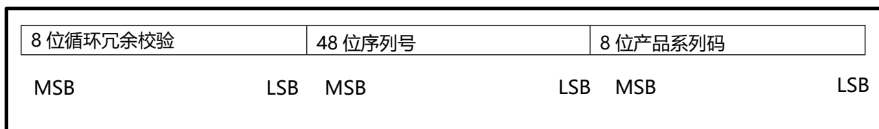
图 10.1 64 位 ROM 编码
