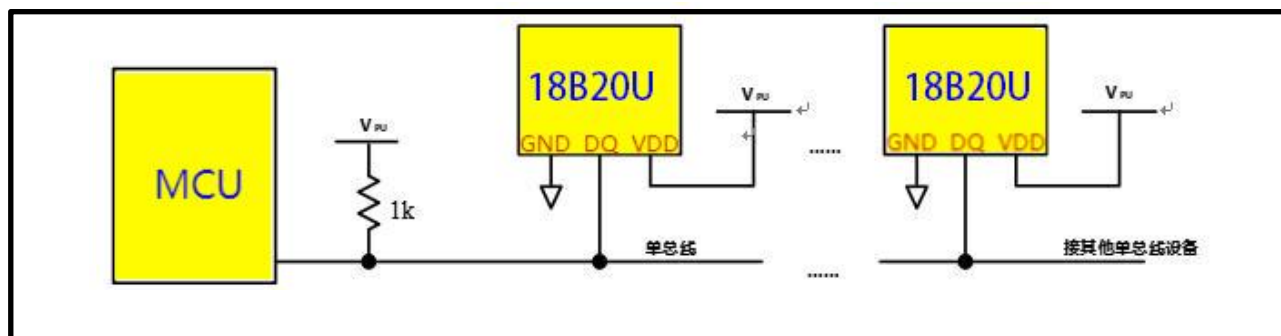
图 9.1 外部供电模式示意图
