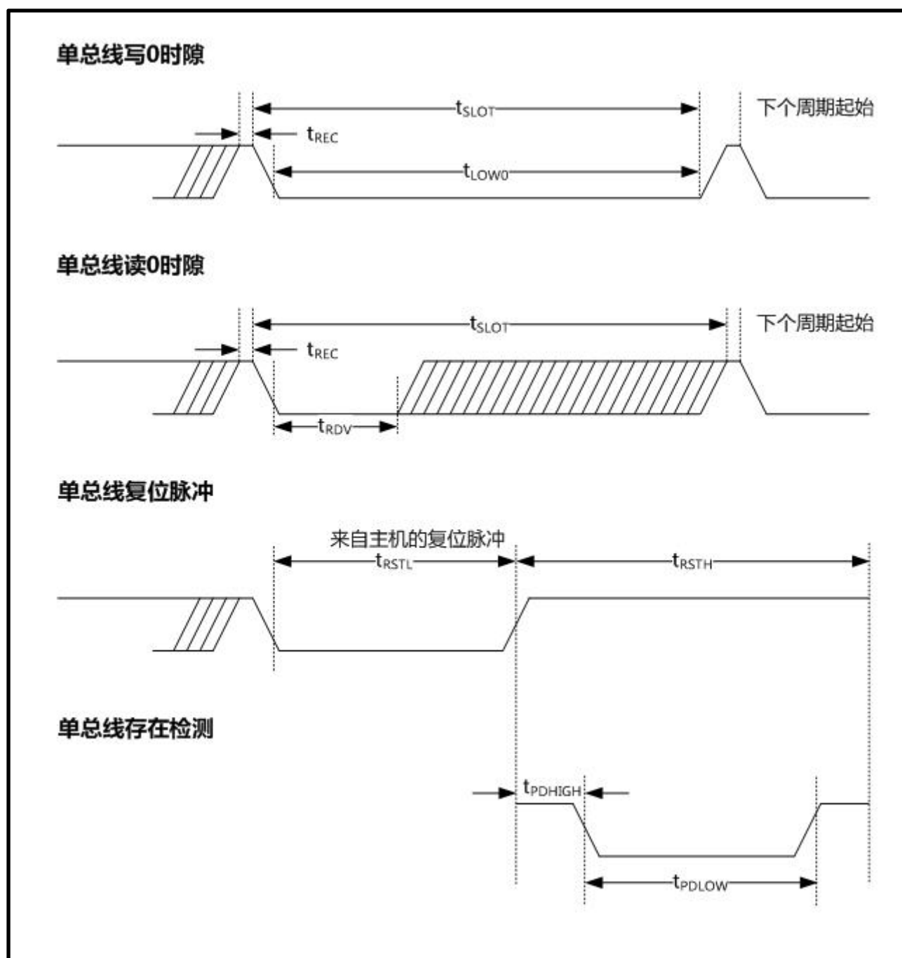
图 11.6-5 时序图
