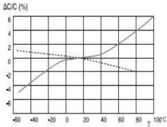
容量与温度曲线图
