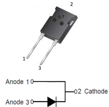
TO247-2L
