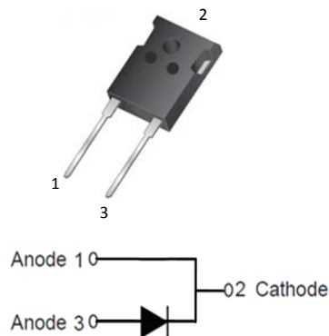
TO247-2L
