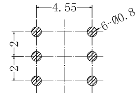
PCB参考图
