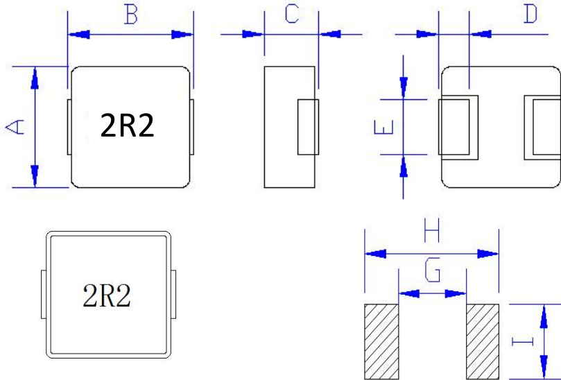
压边外形
