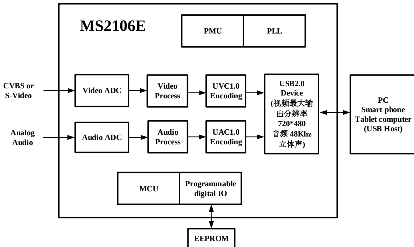
图一. MS2106E 功能框图
