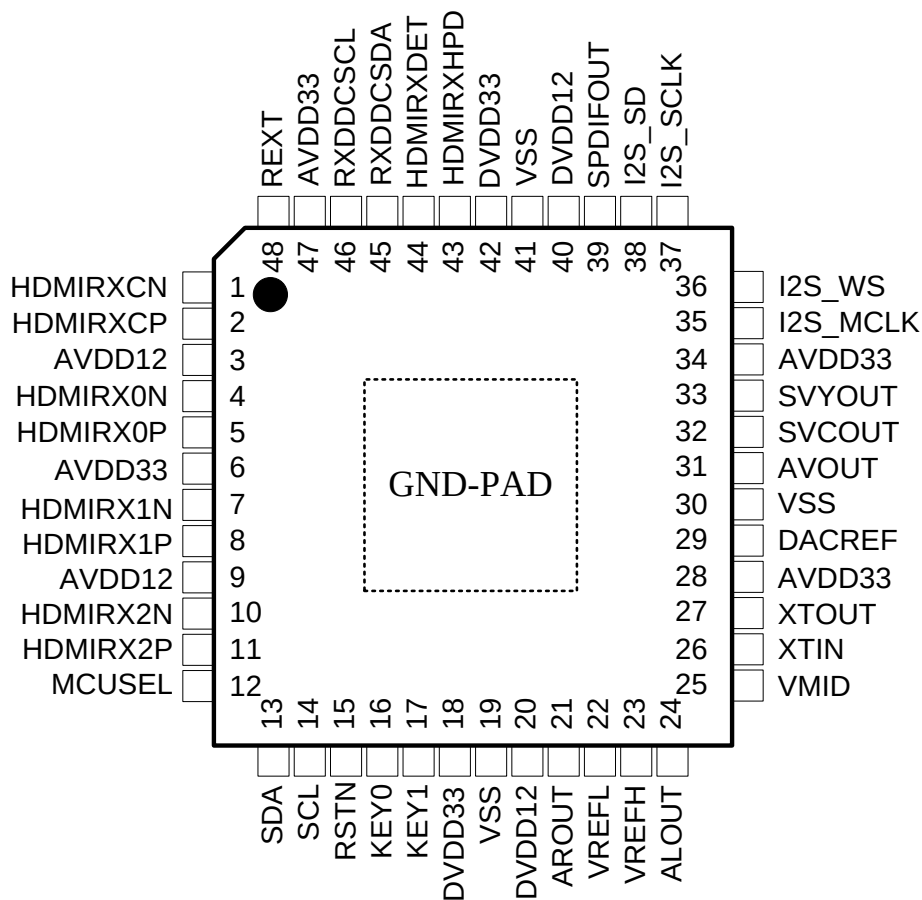
图二. 引脚图
