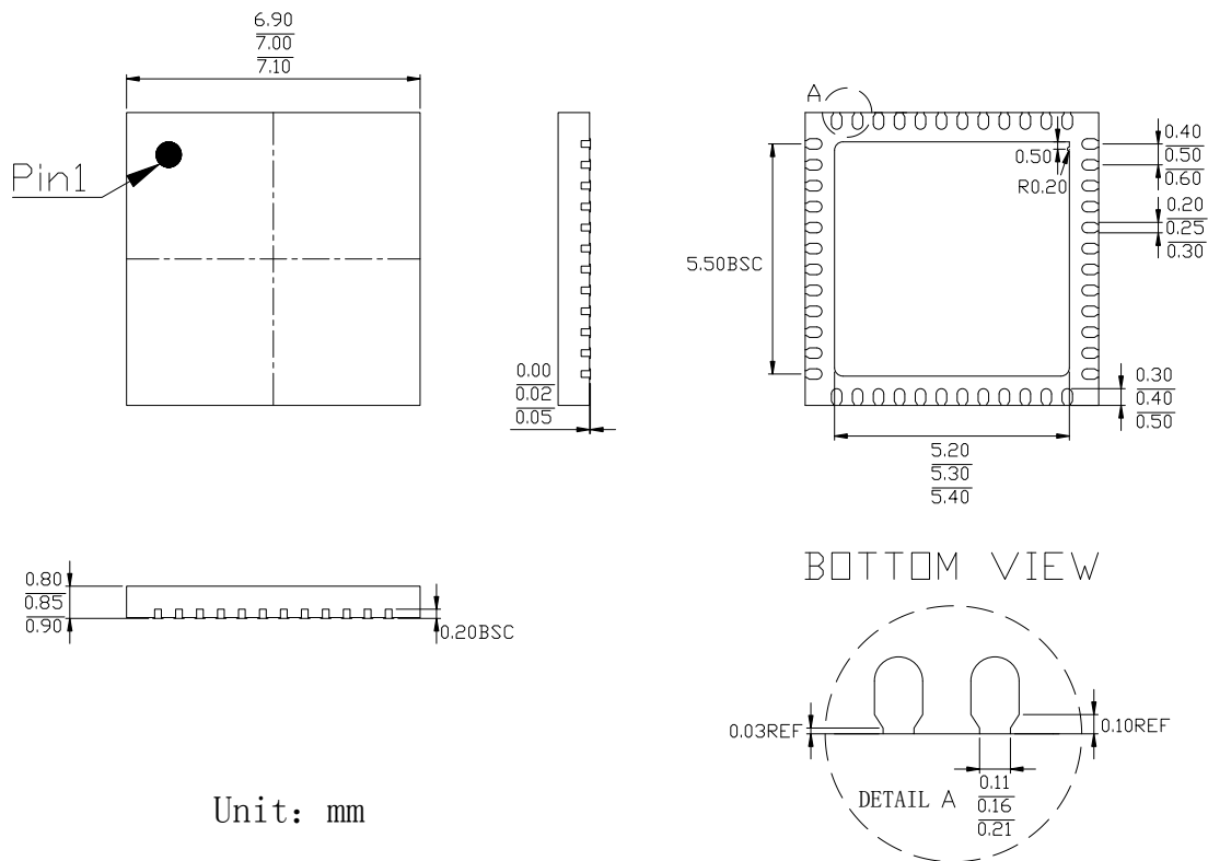
图四. QFN48 封装框图
