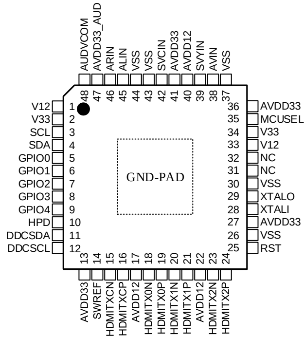
图二 MS1858E 引脚图
