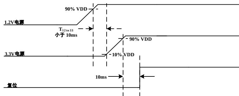
图六. 上电时序
