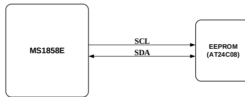
图四. 内部主控模式
