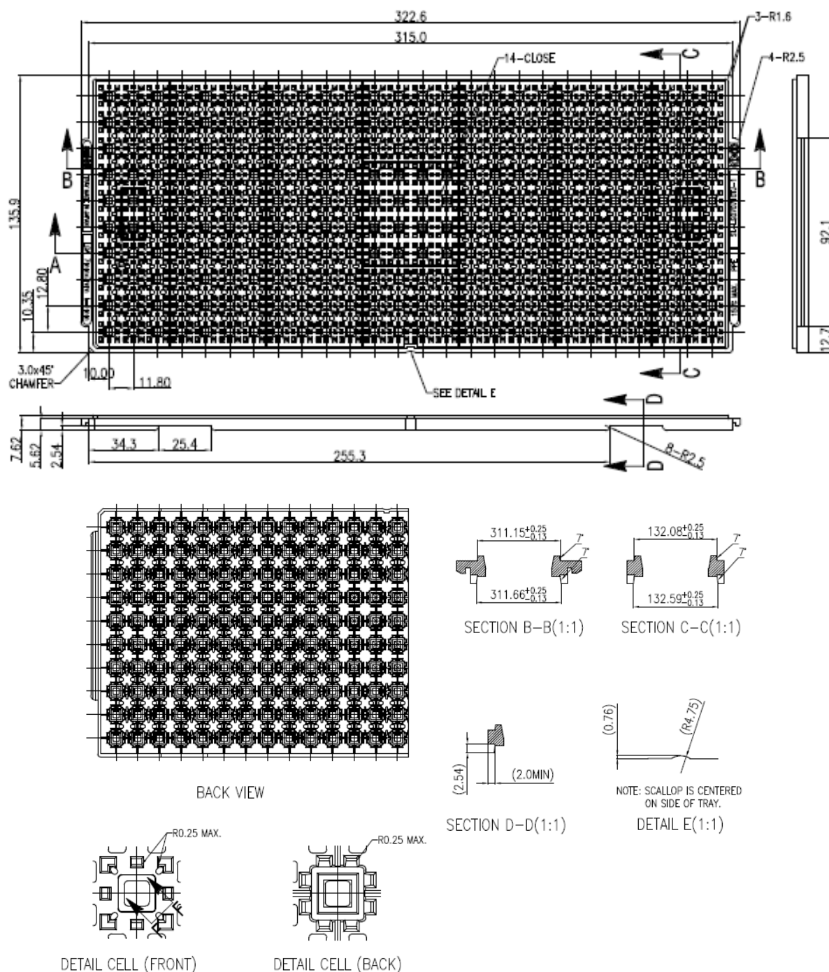
图十. 托盘尺寸信息
