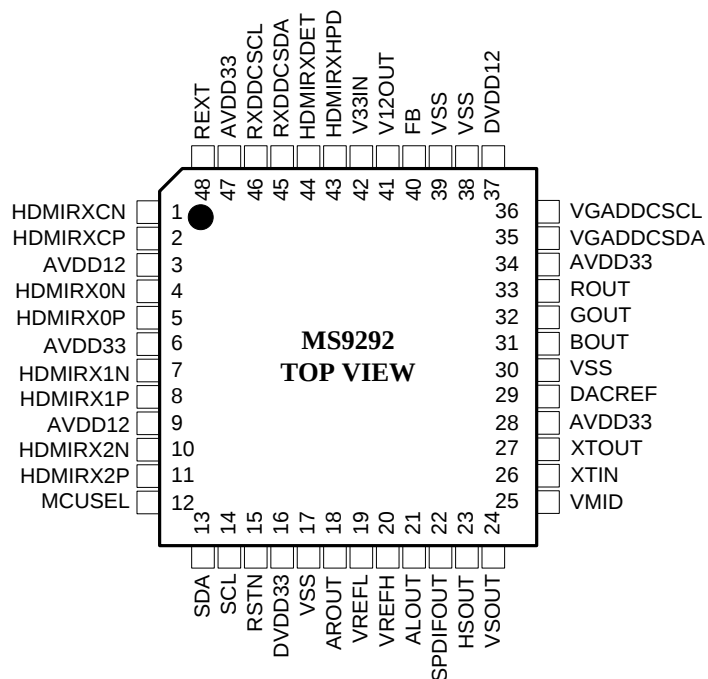
图二. 引脚图
