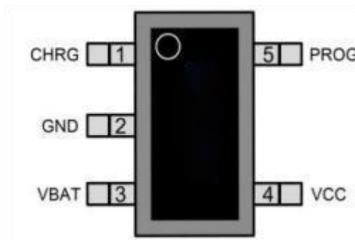
SOT23-5L
