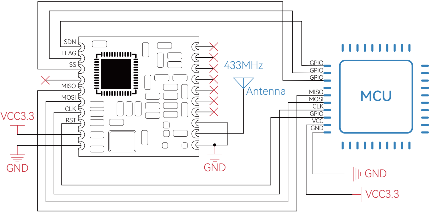
正常使用GP0、GP1、GP2、GP3可不接，其中NC为内部悬空脚可不接
