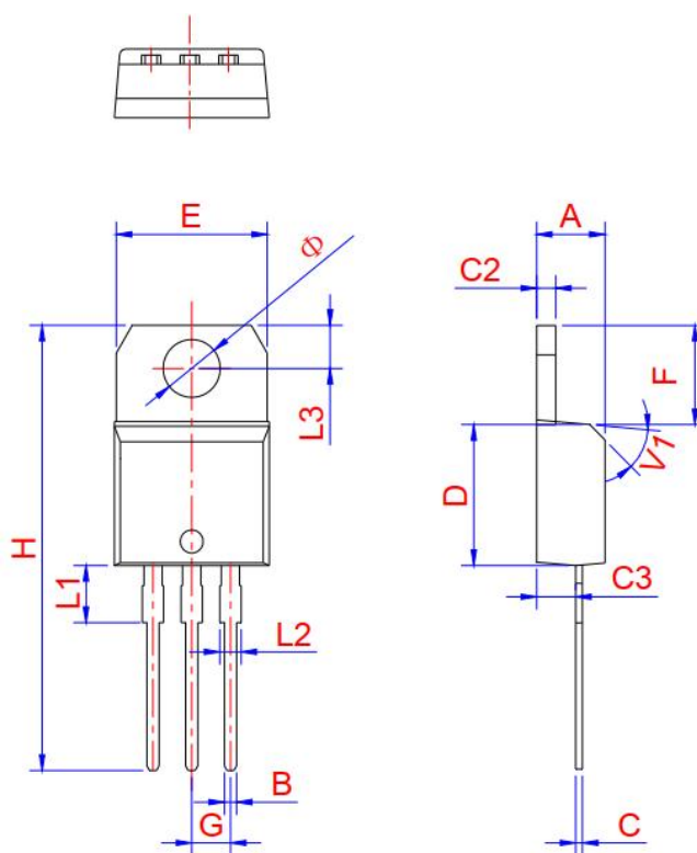
TO-220A Ins
