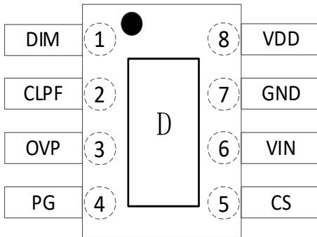
图 5 Hi150XE 管脚图
