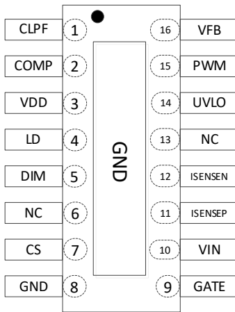
图 5.2 Hi5000 管脚图
