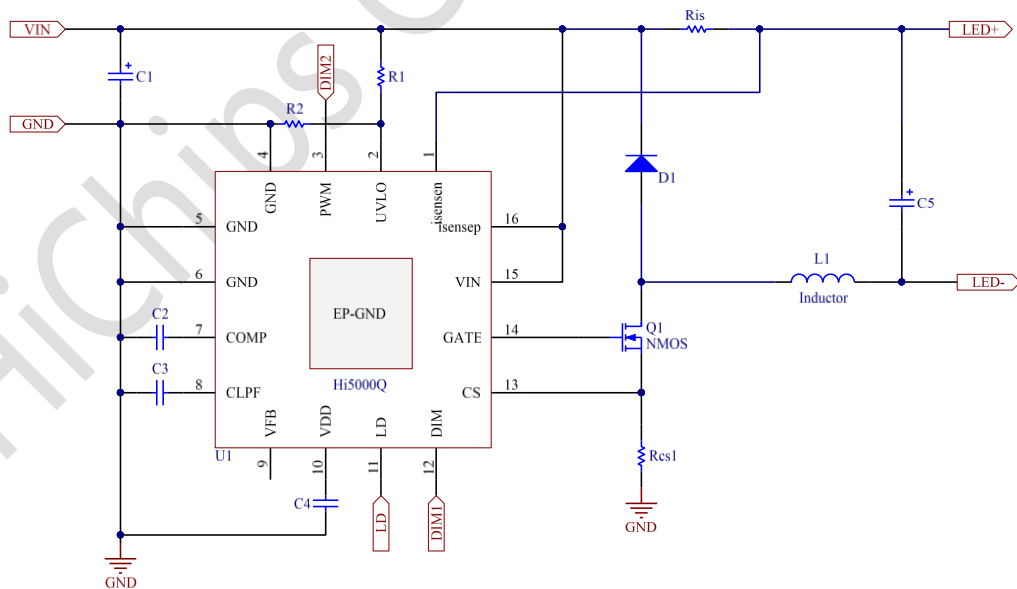
图 7.2 典型应用电路——降压不共阳接法
