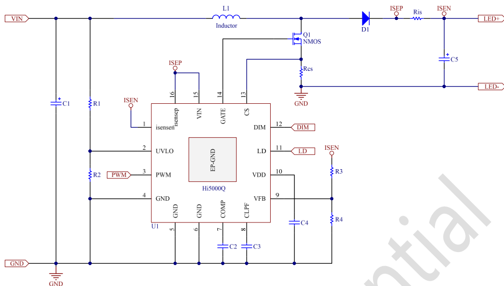
图 7.3 典型应用电路——升压接法
