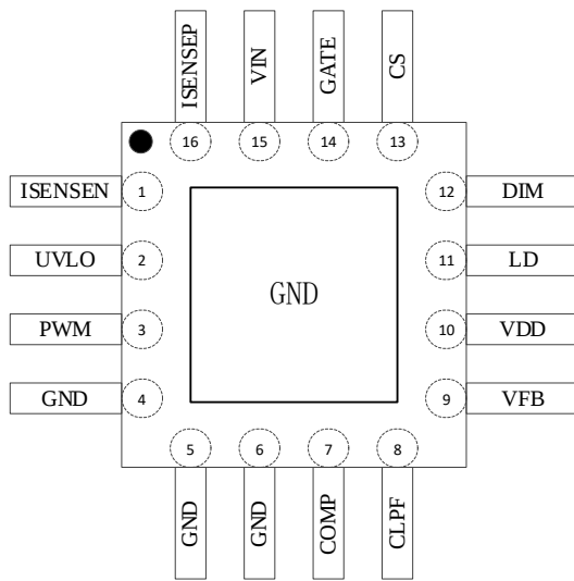
图 5.1 Hi5000Q 管脚
