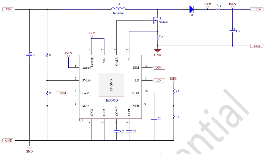
图 8.3 典型应用电路——升压接法
