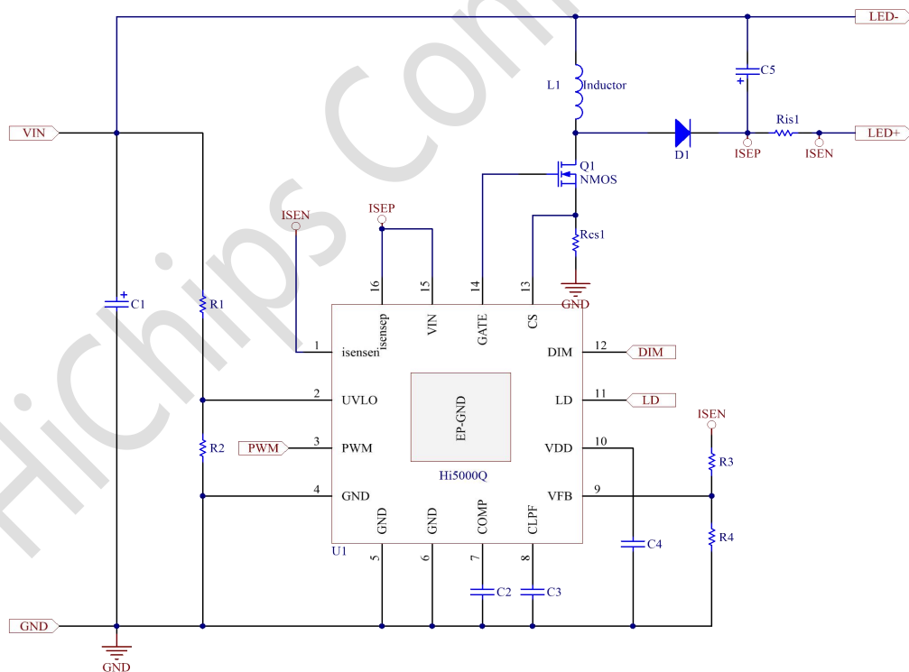
图 8.4 典型应用电路——升降压接法
