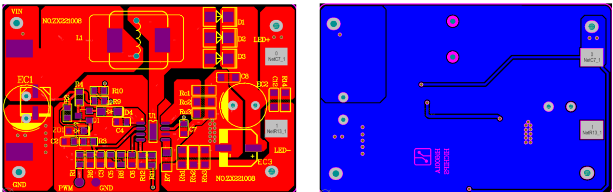
PCB 图
