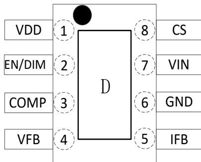
图 5.1 管脚图
