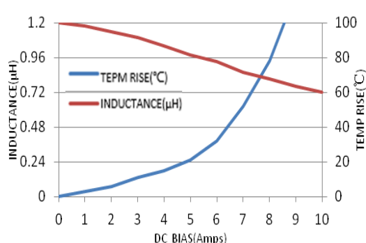
FSA0420-1R2MT
