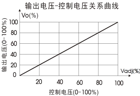
图 3 输出电压与控制电压关系曲线
