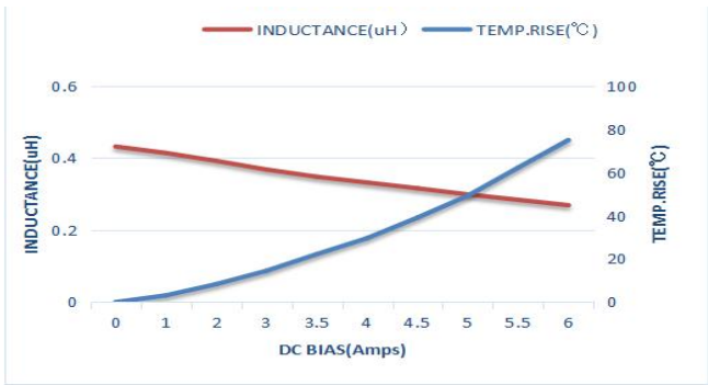
AFE141208SR47MBT
