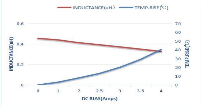
AFE141265SR47MBT
