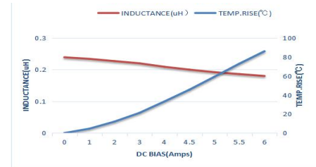
AFE160808SR56MBT
