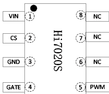
图 5-1 Hi7020S 管脚图
