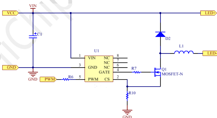
图 4-1 Hi7020S 应用电路
