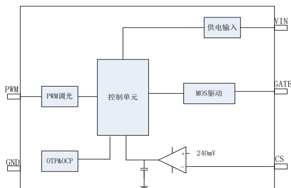
图 7-1 结构框图
