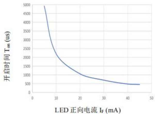
图.10 开启时间-正向电流特性
