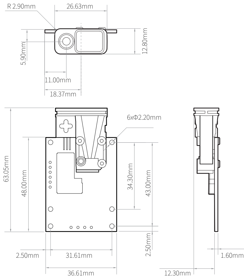
图 5. L2 尺寸图
