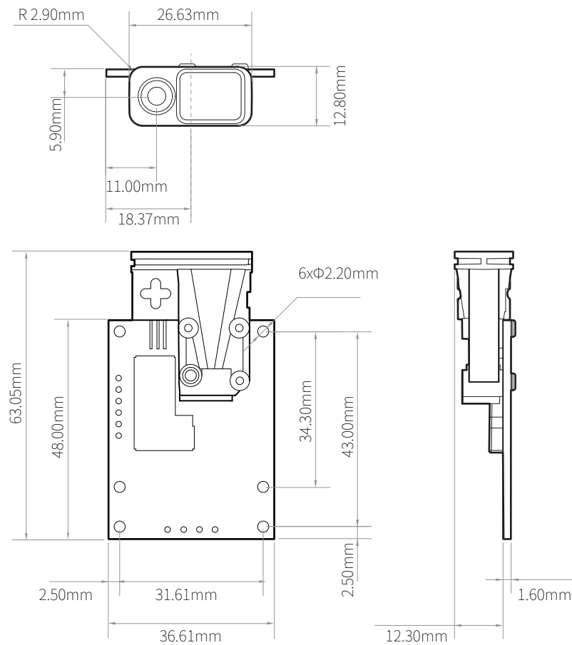
图 5. L2 尺寸图
