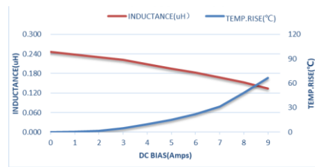
AFE201208SR68MBT
