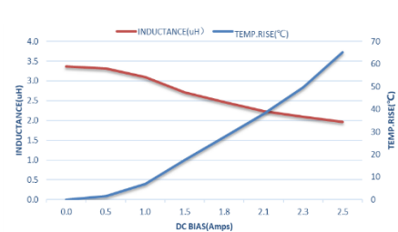
AFE201208S3R3MBT
