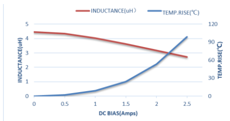
AFE201212SR11MBT
