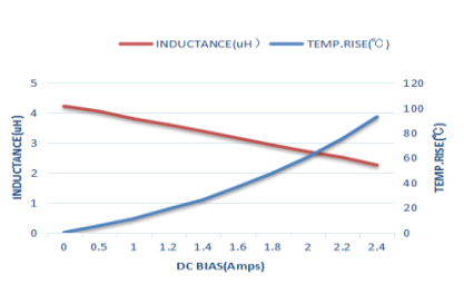
AFE201208S4R7MBT
