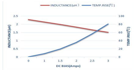
AFE201208S2R2MBT
