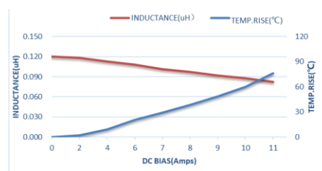
AFE201208SR24MBT
