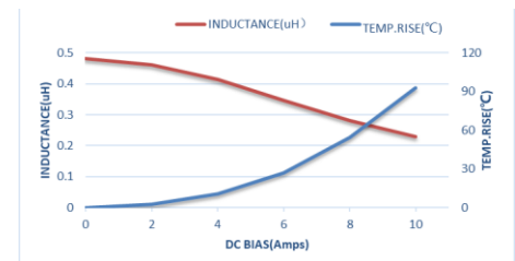
AFE201212SR47MBT
