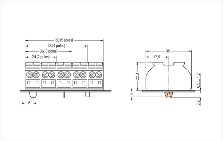
外形尺寸 (单位 : mm) 外形尺寸(单位 : mm) 用于小型接线端子排
