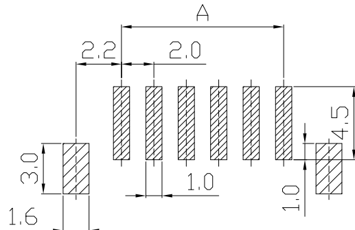
PCB 参考图
