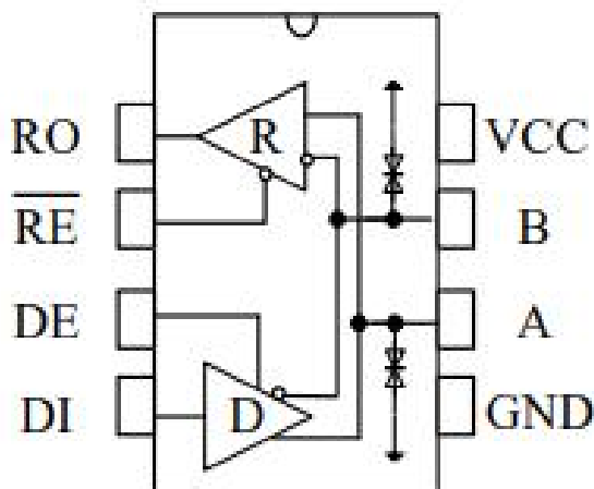
图 1 SSP485 引脚分布图
