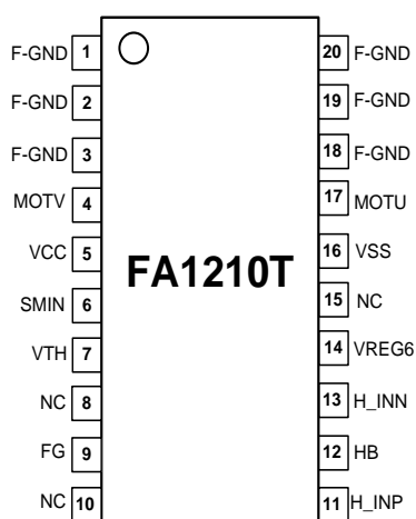
TSSOP20
