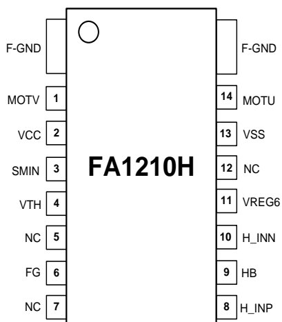
HTSSOP14
